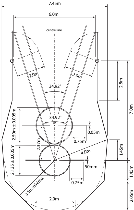
Figura 24.- Jaula para el Lanzamiento de Martillo y Disco con círculos independientes
